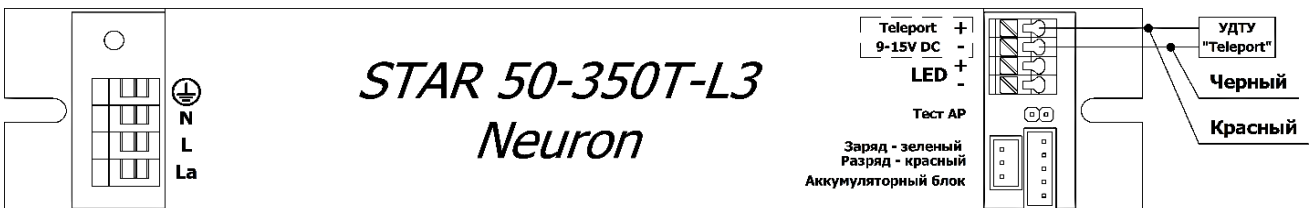
Рисунок 11 – Схема подключения УДТУ «Teleport»
