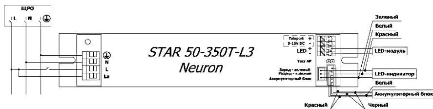
Рисунок 9 – Схема подключения БАП
