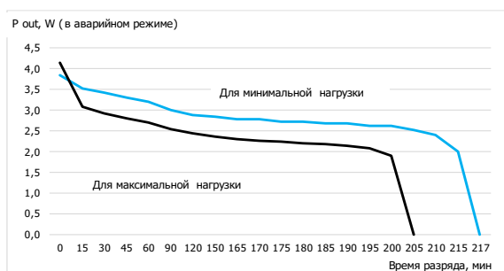
Рисунок 8 – Зависимость мощности в аварийном режиме от времени разряда (на max и min нагрузке)
